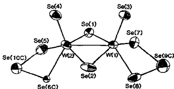
Fig. 25. The W_2Se_4(Se_3)_2^{2-} ion [20].
